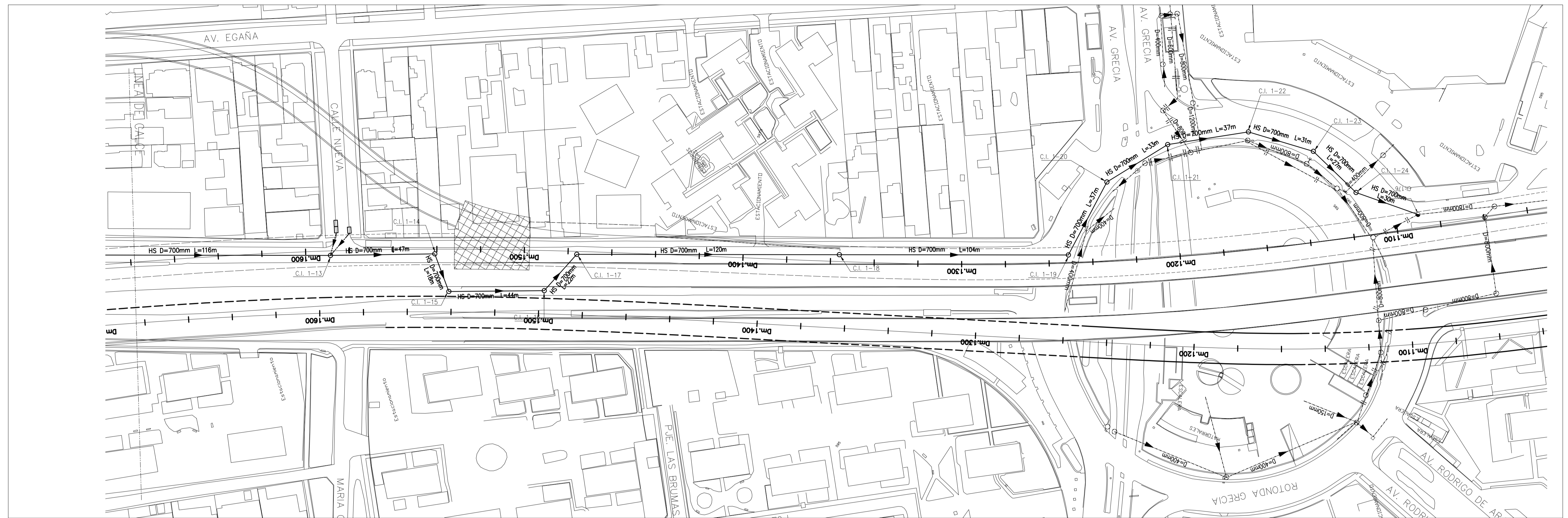
PLANTA COLECTOR N°1 ESCALA 1:1000
